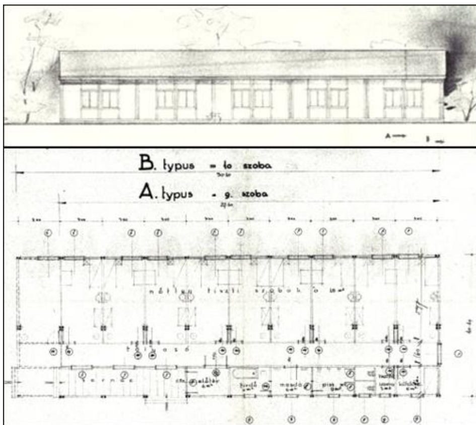
8. ábra A nőtlen tiszti lakások látképe és alaprajza
