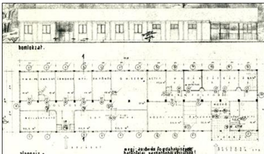
5. ábra A. típusú iroda űr-fogda épület látképe és alaprajza Forrás Hadtörténelmi Levéltár
