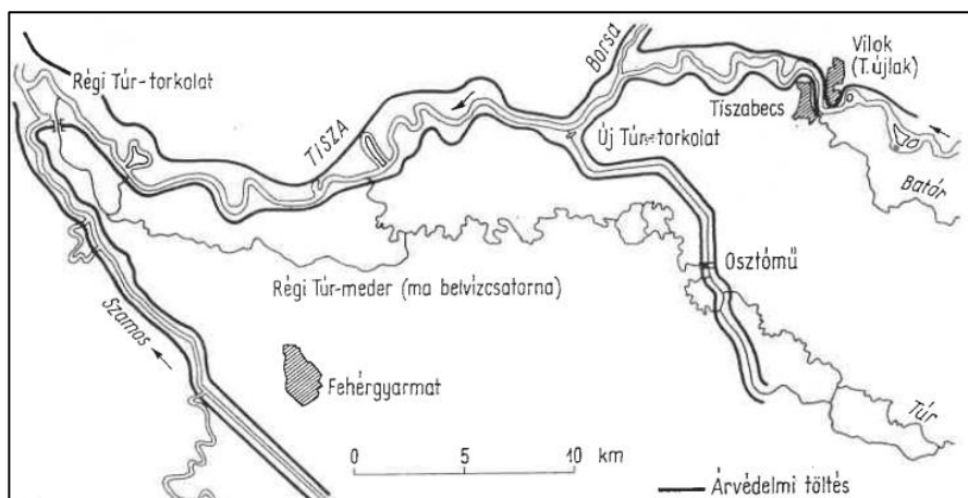
6. ábra. A Túr folyó medervonalai
