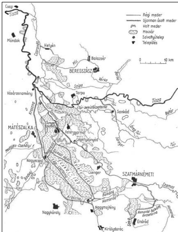
7.ábra. A Kraszna és a Tisza-Szamos-köz szabályozása
