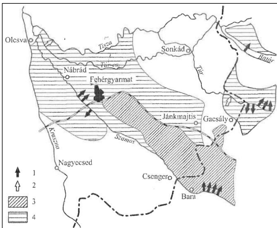
5. ábra. A Szamosvölgyi árvíz térszerkezete
