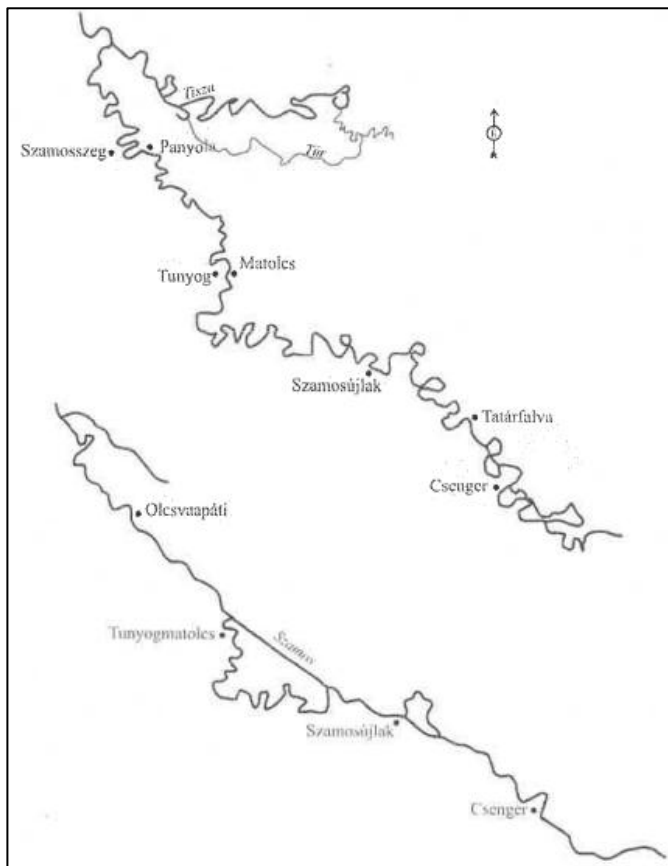
4. ábra. A Szamos jellemző mederformái az 1770-es és az 1860-as évek között
