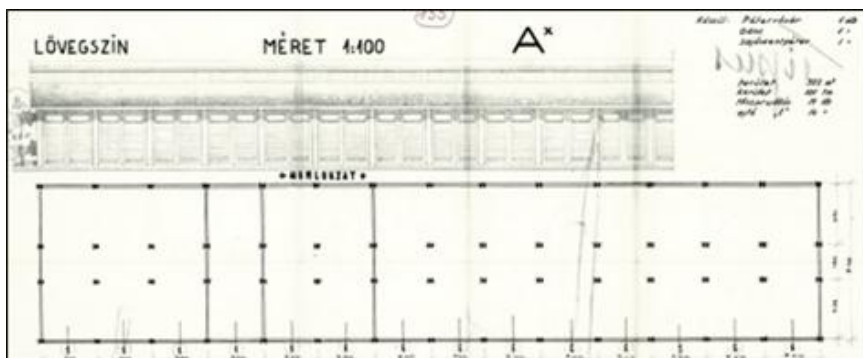
6. ábra C. típusú lövegszín látképe és alaprajza Forrás Hadtörténelmi Levéltár
