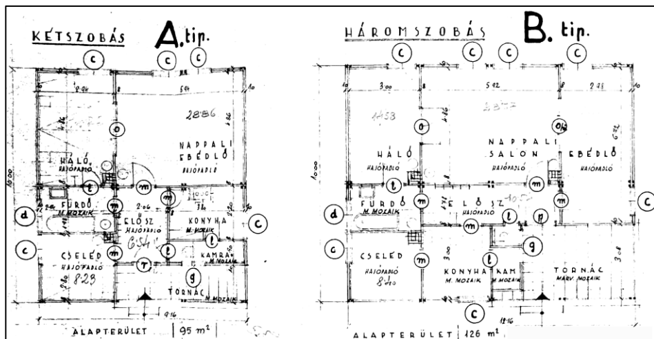
9. ábra Tiszti lakástípusok alaprajza
