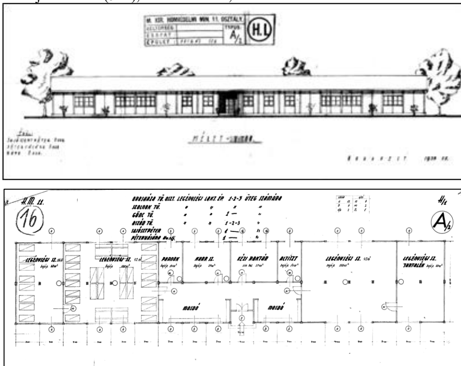
4. ábra A/2 légénységi barakk látképe, alaprajza Forrás Hadtörténelmi Levéltár
