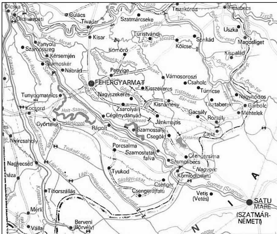
2. ábra. A Szatmári-síkság vízhálózata
