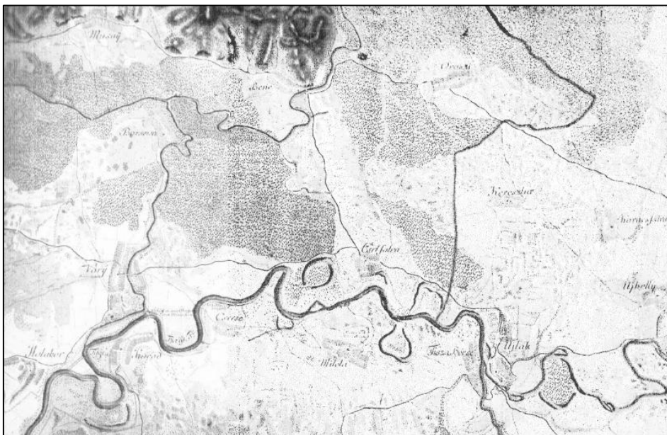
3. ábra. A Tisza medervonala a szabályozása előtt Tiszabecs-Tiszacsécse között
