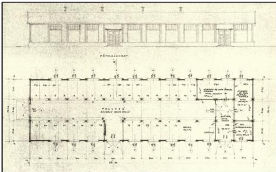
7. ábra A/32 típusú istálló látképe és alaprajza Forrás Hadtörténelmi Levéltár
